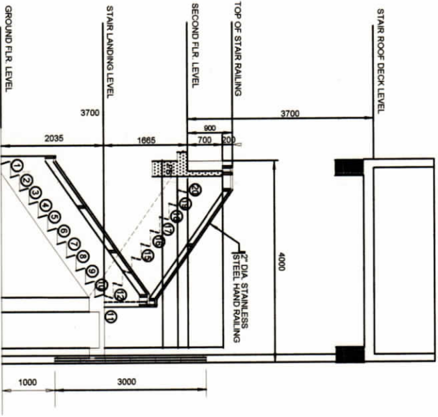
3 ELEVATION A-3 SCALE 1 : 60 M.
